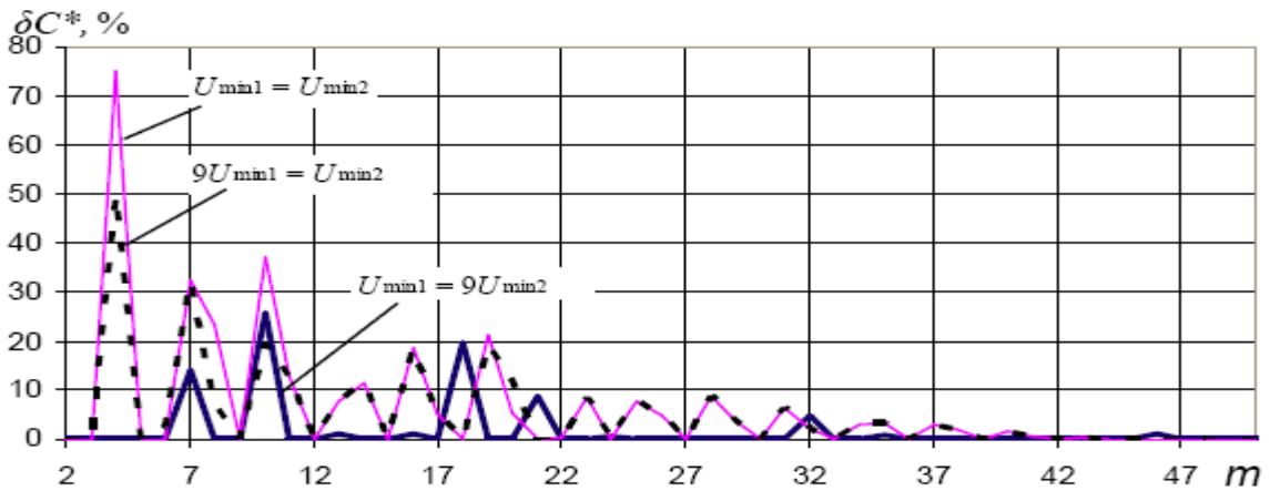
Fig. 4.7. Dependența indicatorului relativ \delta C^* de numărul m de tipuri de servere și structura fluxului total de cereri la U_{\min} = 10 Gflops.
